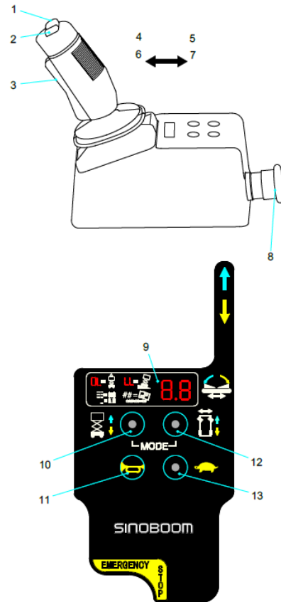
Abbildung 6-3 Plattformbedienpult (DTC)
