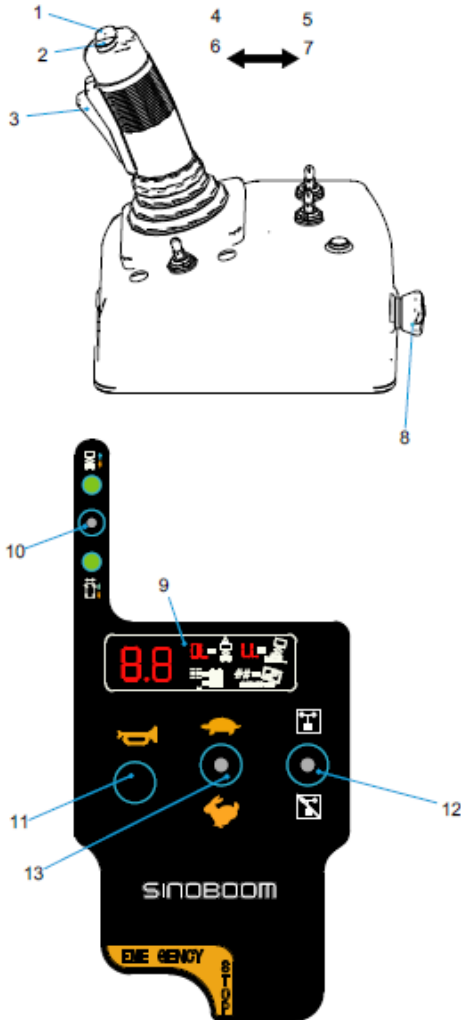
Abbildung 6-2 Plattformbedienpult (SINOBOOM)
