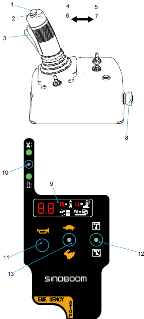
Abbildung 6-2 Plattformbedienpult (SINOBOOM)
