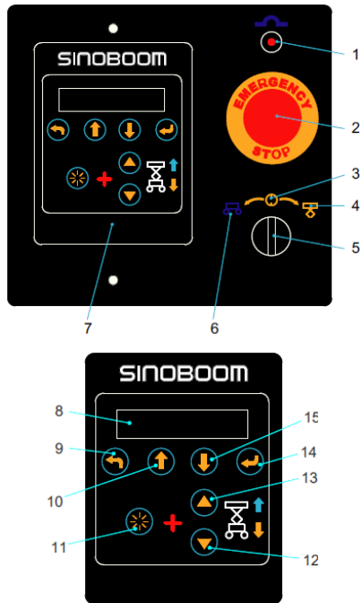
Abbildung 6-1 Bodenbedienpult
