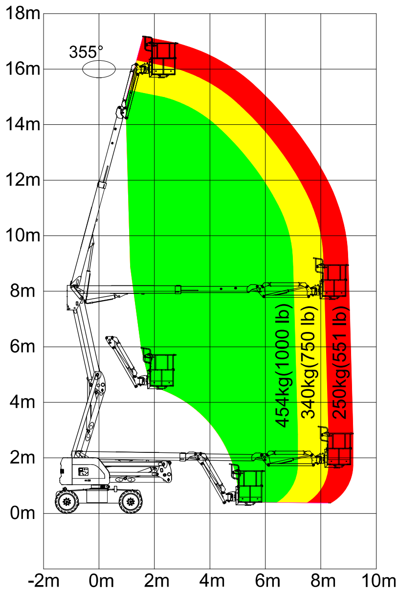
Fig 1 Diagramm: Arbeitsbereich (-5°)
